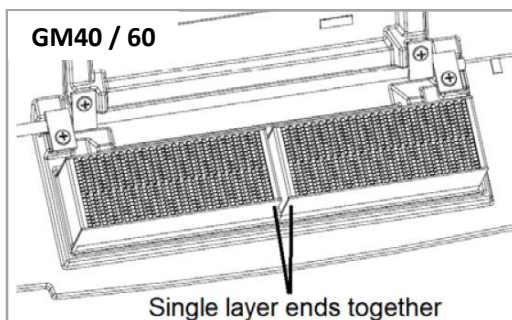
図 10. コンバスターの収め方 （※ガスケットを巻いた場合のみ）1重に巻いた短辺が中央で隣り合うように収めてください。
