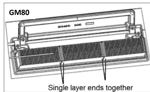
図 10. コンバスターの収め方 （※ガスケットを巻いた場合のみ）1重に巻いた短辺が中央で隣り合うように収めてください。
