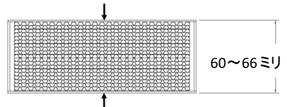
図 8. コンバスター:寸法の見方
